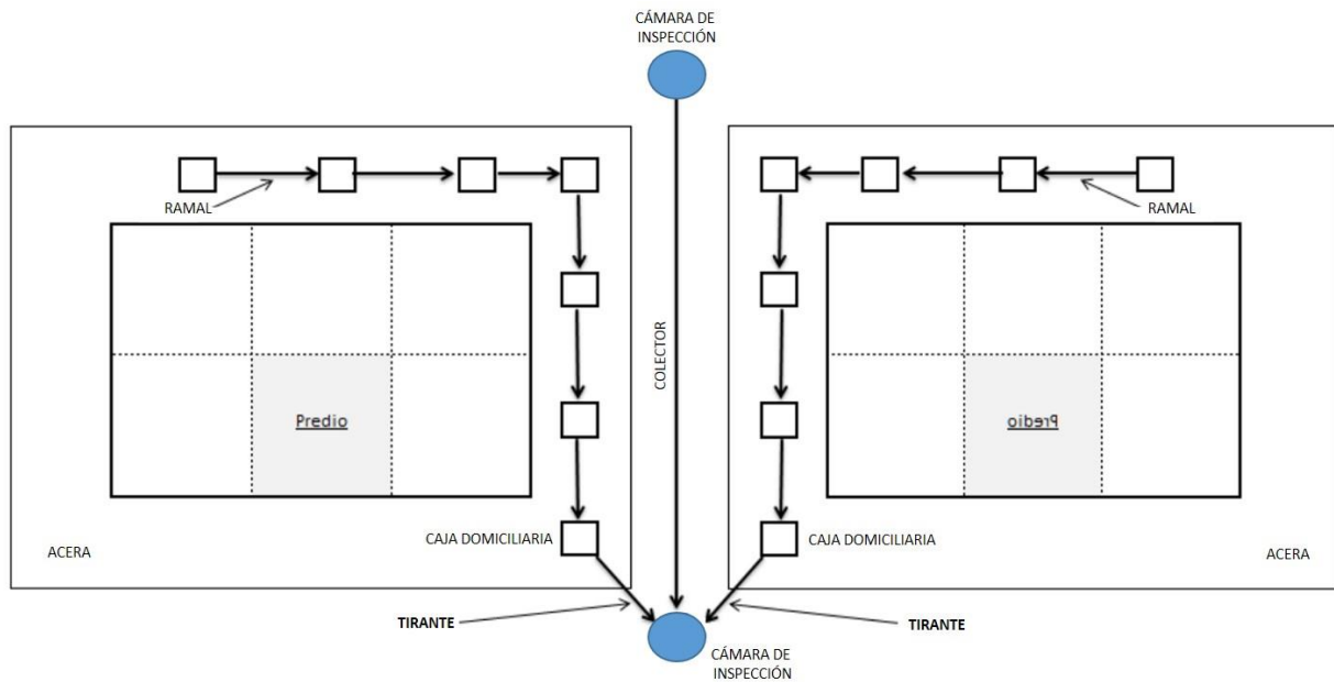
Configuración Típica de la Red de Alcantarillado Sanitario de Guayaquil
