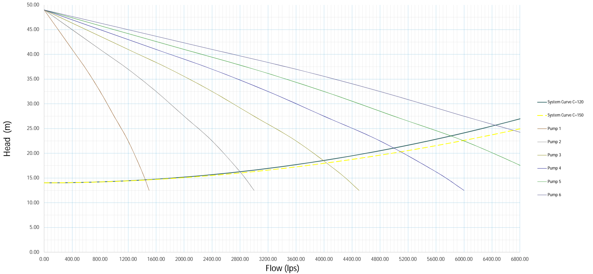
Estacion de Bombeo Pradera 4200-6400 Ips Flygt Model CT-3531/ 905 / 620 mm Impeller, 450 HP @ 890 RPM
