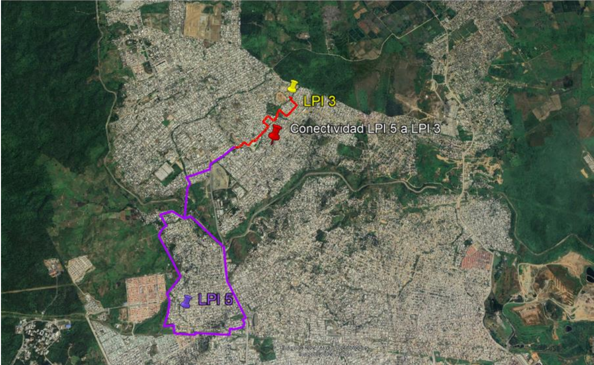
Figura 2. Esquema Conectividad LPI 5 a LPI 3 (en color rojo colector a gravedad previsto ejecutar).
