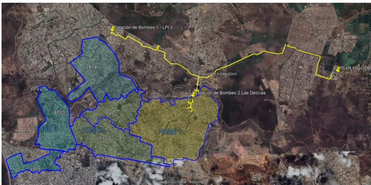
Figura 1. Esquema área de influencia Sistema 3 de Alcantarillado Sanitario en el noroeste de la ciudad de Guayaquil.
